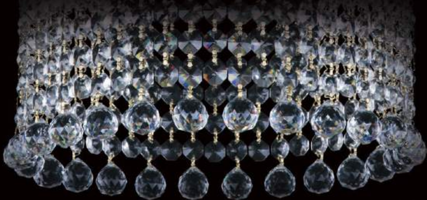
21.201.25SP.G.Dr ↔ 25 cm † 26 cm 💡 x 3 (E14 - 40W) weight ≈ 3 kg
