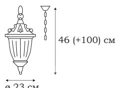
■ L79001.12 1 x E27 (100W), IP - 43
