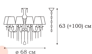
■ L19910.09 10 x E14 (40W)
