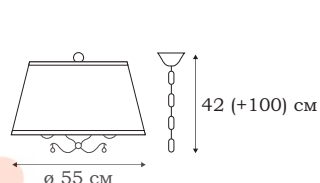
■ L17805.03 5 x E14 (60W)
