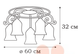
■ L17755.19 5 x E27 (60W)
