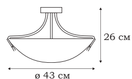
■ L13053.88 3 x E27 (60W)
