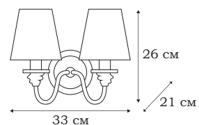
■ L12222.02 2 x E14 (60W)
