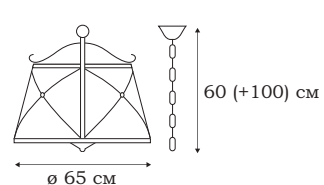
■ L57705.08 5 x E14 (60W)
