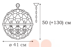
■ L51104.68 4 x E14 (60W)
