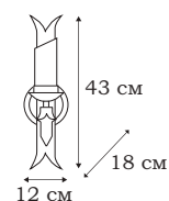
■ L16921.04 1 x E14 (60W)
