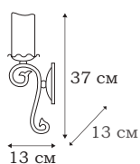
■ L13821.03 1 x E14(60W)
