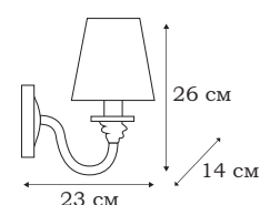
■ L12221.37 1 x E14 (60W)
