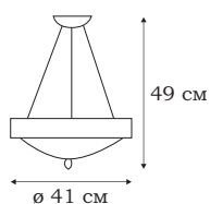
■ L14804.89 4 x E14 (60W)
