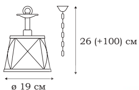
■ L12101.88 1 x E14 (60W)
