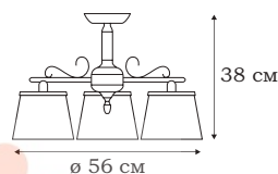
■ L12153.88 3 x E14 (60W)
