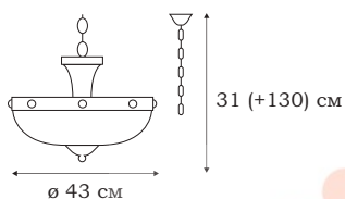
■ L50353.46 3 x E27 (60W)
