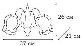
■ L15222.20 2 x E14 (60W)
