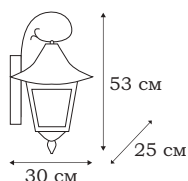
■ L79188.39 1 x E27 (100W), IP - 23
