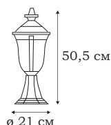
■ L79384.12 1 x E27 (60W), IP - 43
