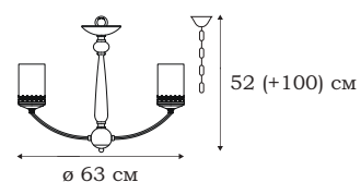
■ L22206.10 6 x E27 (40W)
