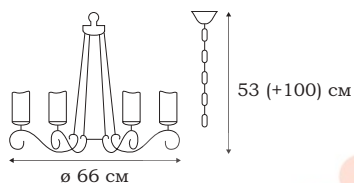
■ L13806.03 6 x E14(60W)
