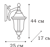
■ L79881.12 1 x E27 (100W), IP - 43
