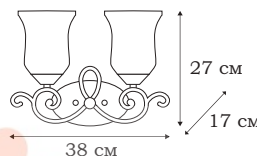
■ L17722.19 2 x E27 (60W)
