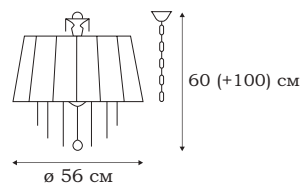
■ L19915.09 5 x E14 (60W)
