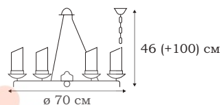
■ L16906.04 6 x E14 (60W)
