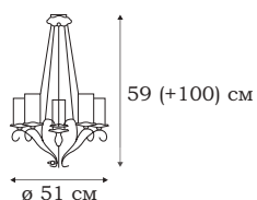
■ L18305.16 5 x E14 (60W)
