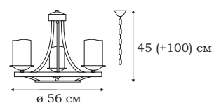
■ L22303.74 3 x E27 (40W)
