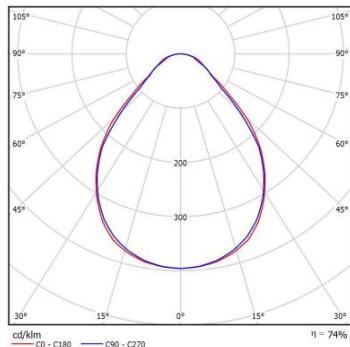
Marenco LED1x1800 A141 T840 ECO
